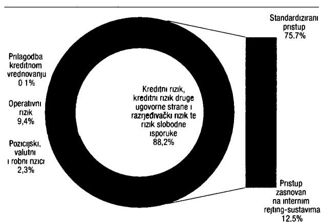
Slika 12.17. Struktura ukupne izloženosti banaka riziku na dan 31. prosinca 2017.
